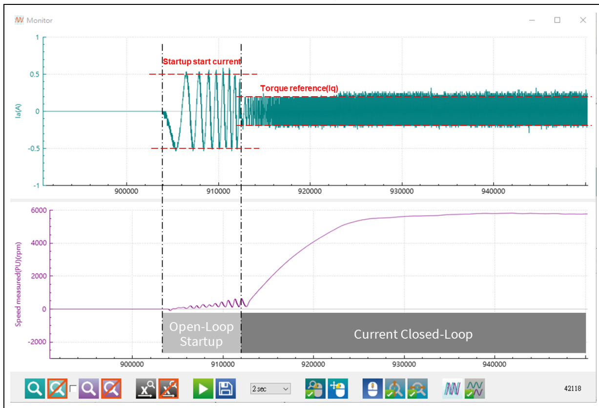
图 40. 电流环控制波形
