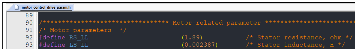
图 11. 电机线圈参数宏定义
