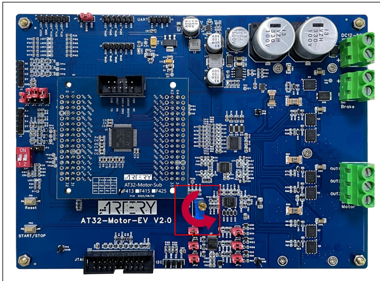
图 50. 电位器位置图 (外部电压控制来源)
