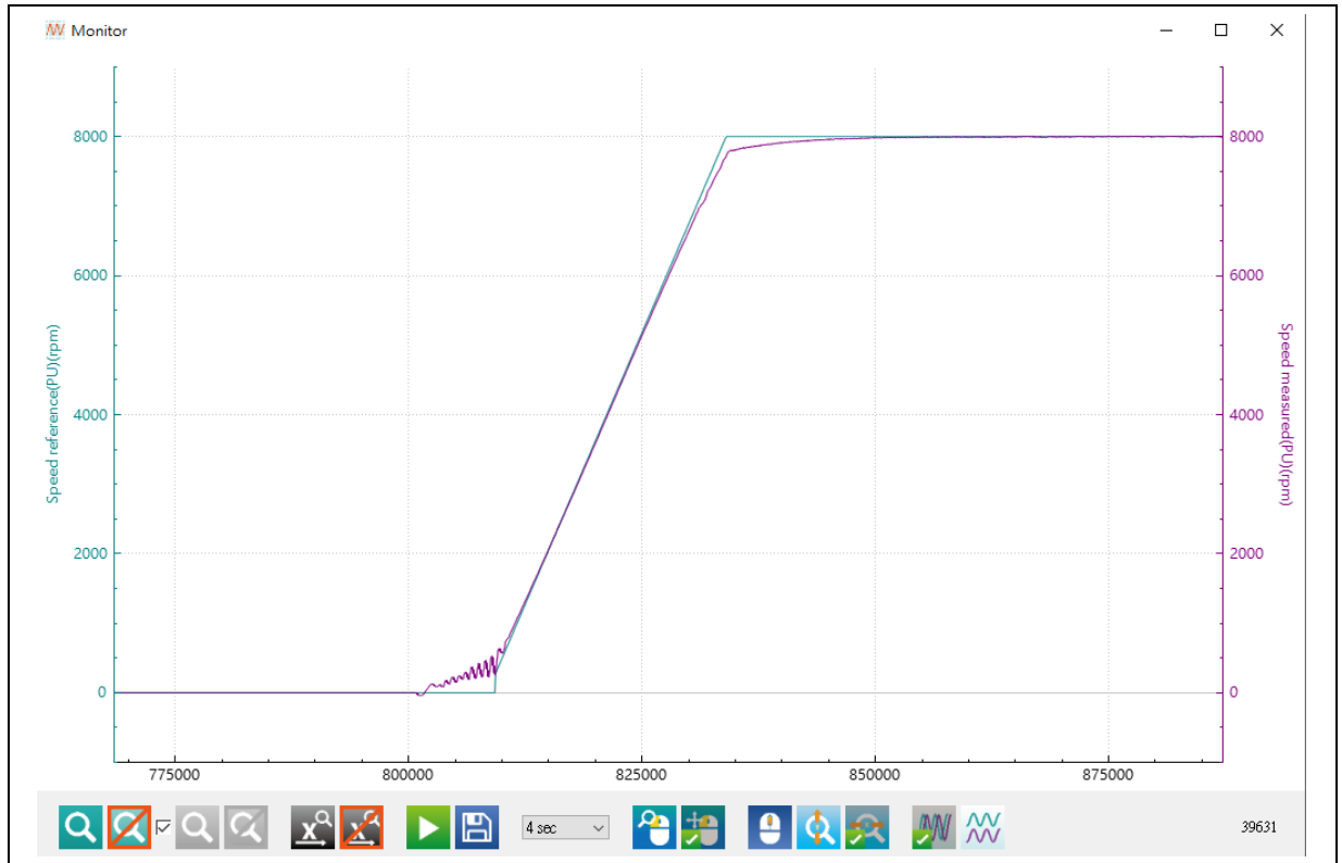
图 48. 速度环(弱磁)调试波形
