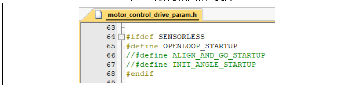
图 26. 无传感器启动方式定义
