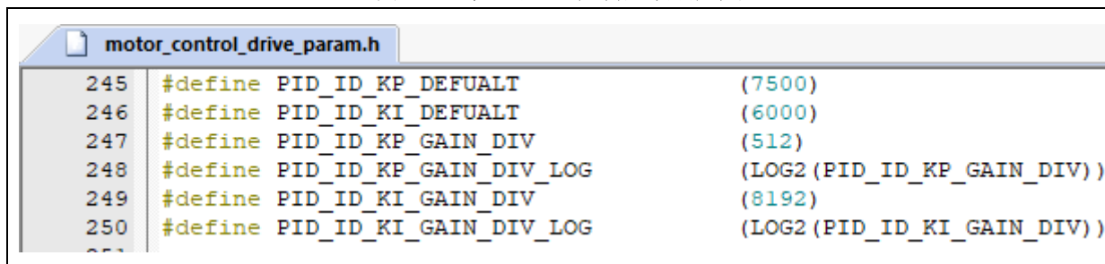
图 20. D 轴电流 PI 控制参数宏定义
