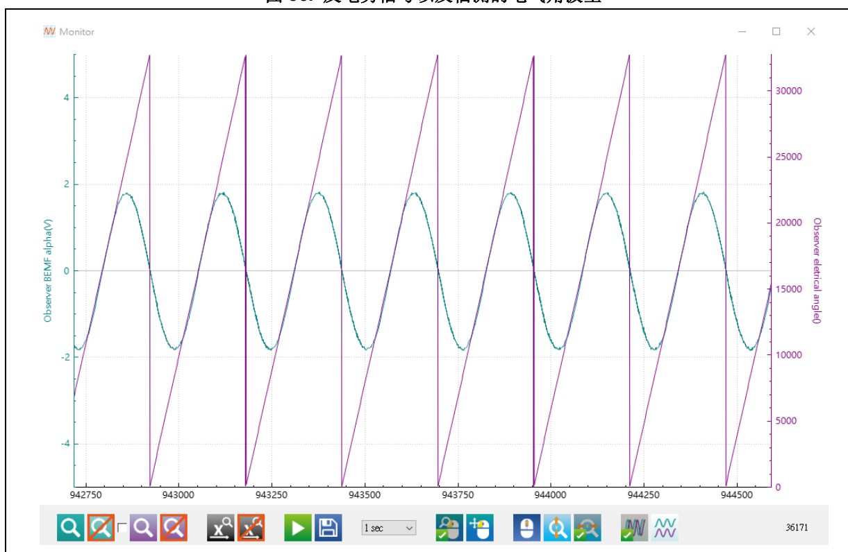
图 36. 反电势信号以及估测的电气角波形
