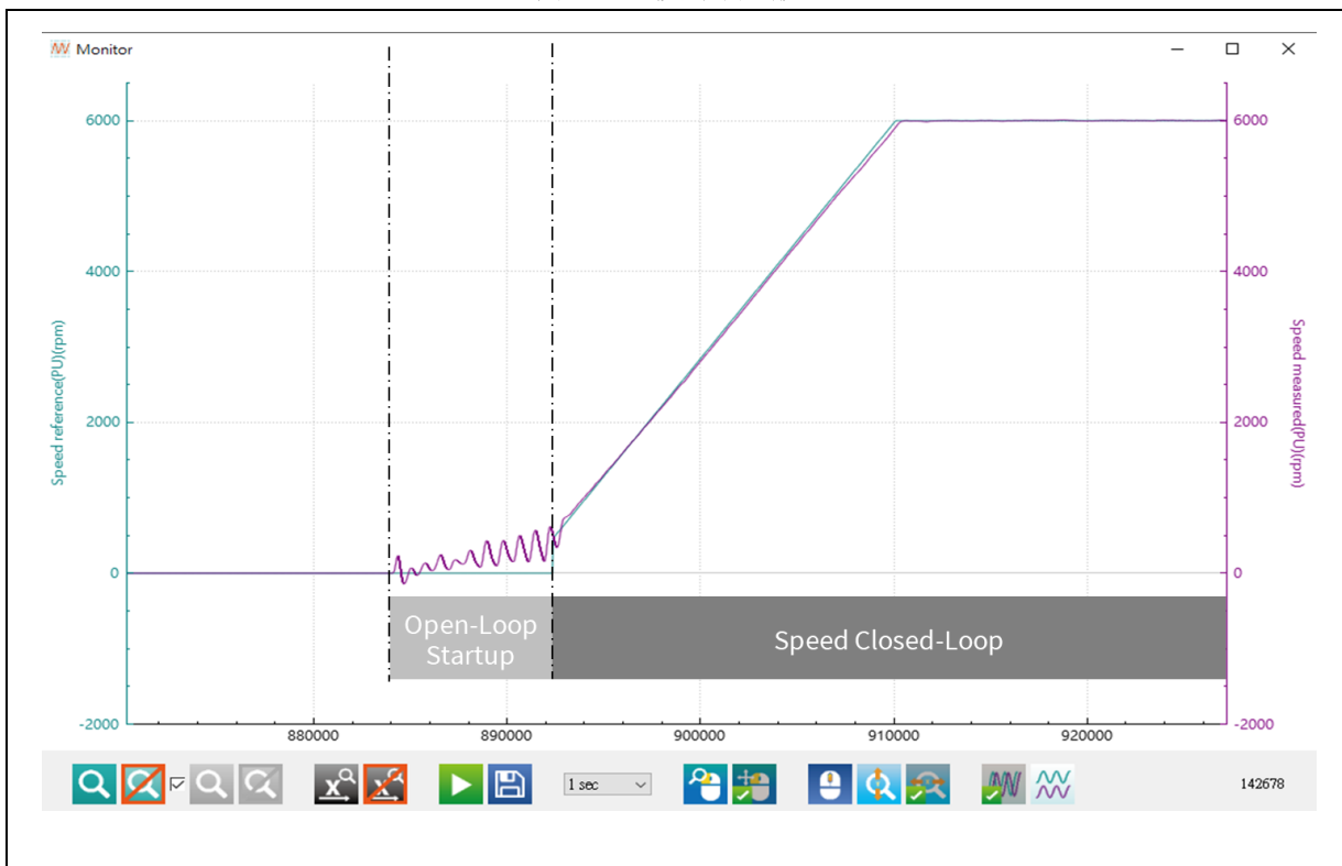
图 44. 速度环调试波形
