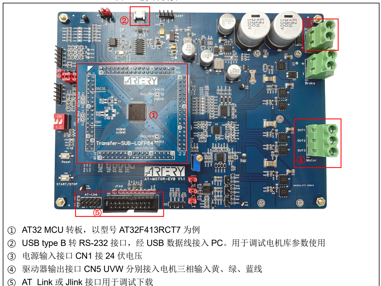
图 1. 电机开发板 AT-MOTOR-EVB V1.x
