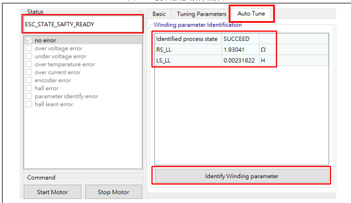
图 10. 电机线圈参数自动辨识
