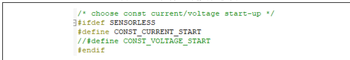
图 27. FOC 无传感器起步方式定义
