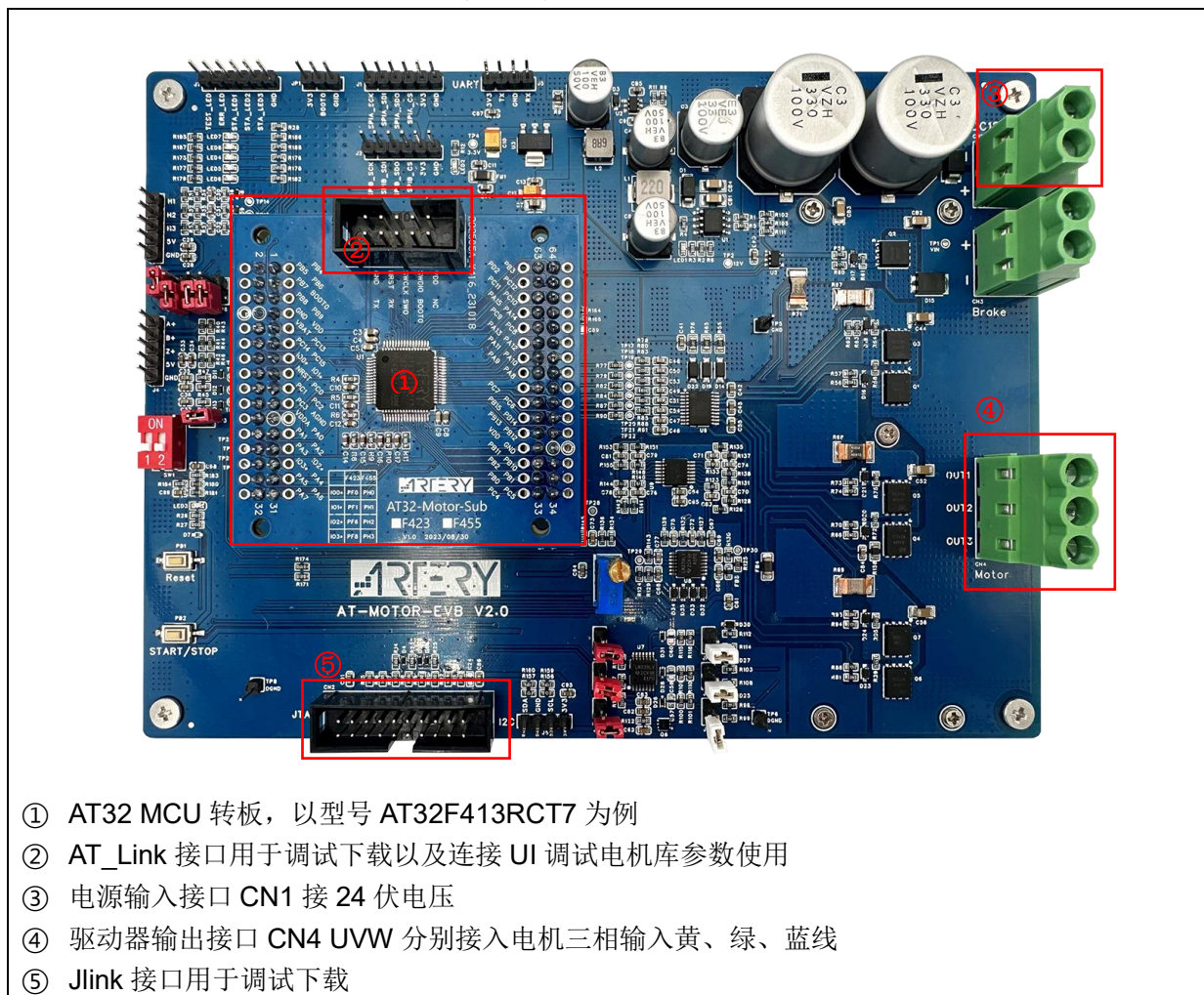
图 2. 电机开发板 AT-MOTOR-EVB V2.x
