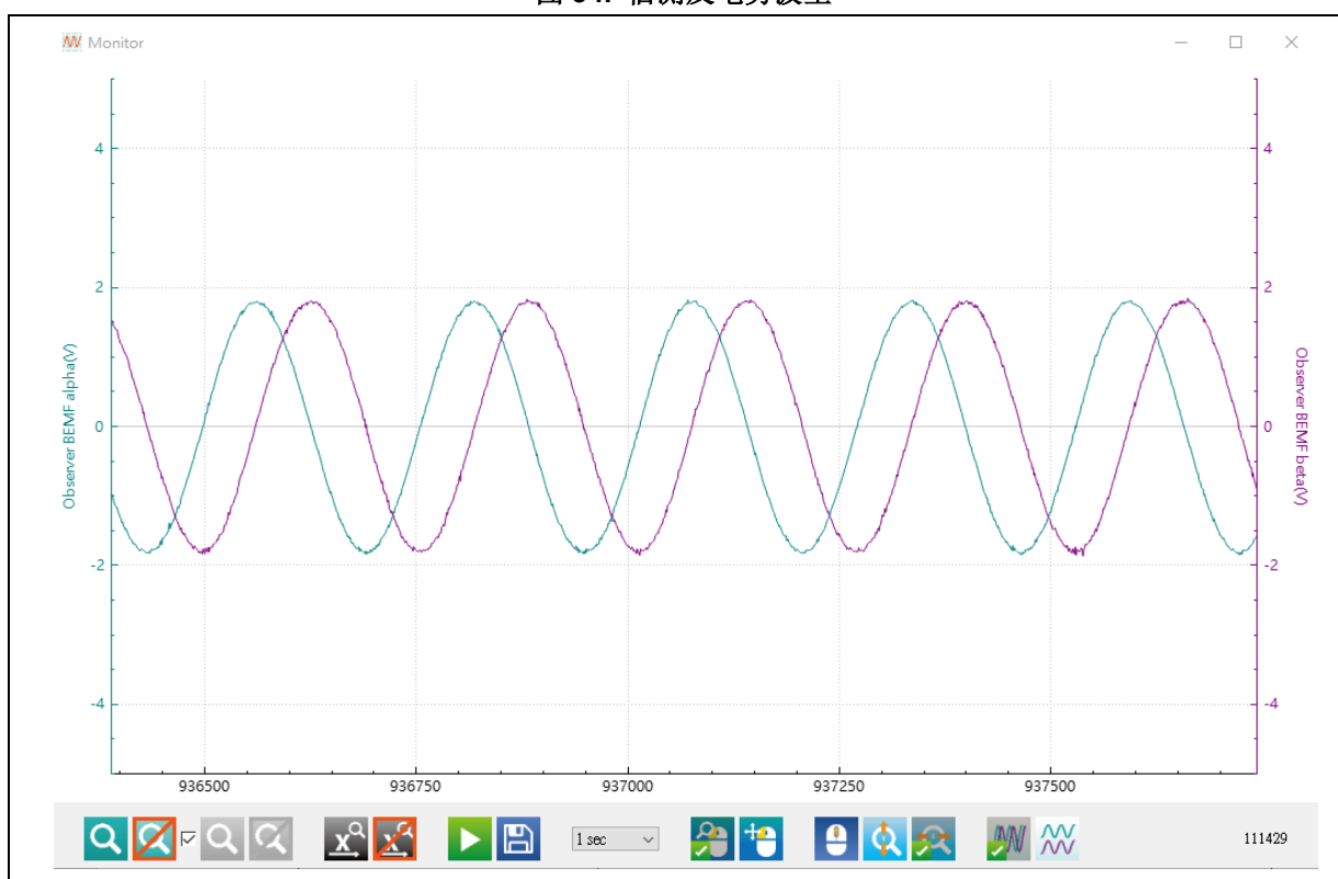
图 34. 估测反电势波形
