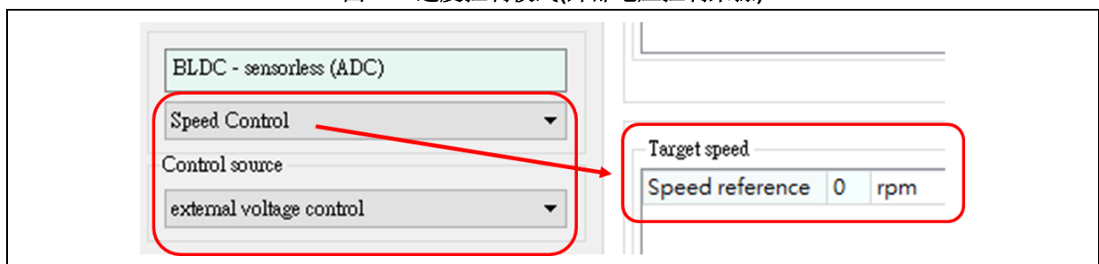
图 52. 速度控制模式(外部电压控制来源)
