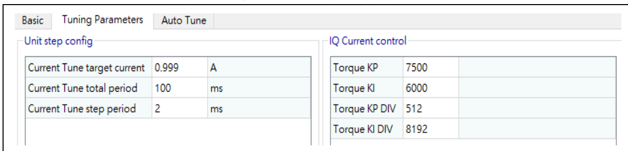
图 22. Q 轴电流 PID 参数以及步阶电流参数
