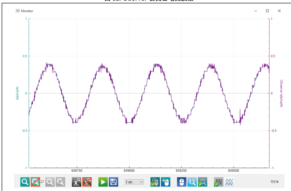
图 32. Observer 估测器电流波形
