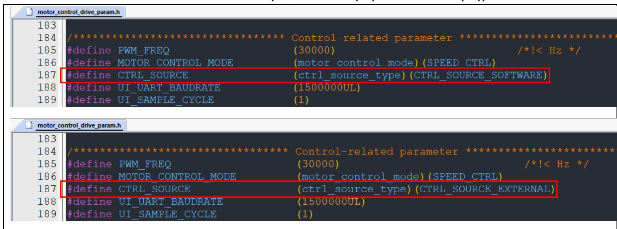
图 51. 控制来源定义值(软件控制来源(上)/外部电压控制(下))
